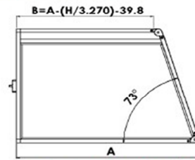
CALCUL DU DÉPORT ARRIÈRE
